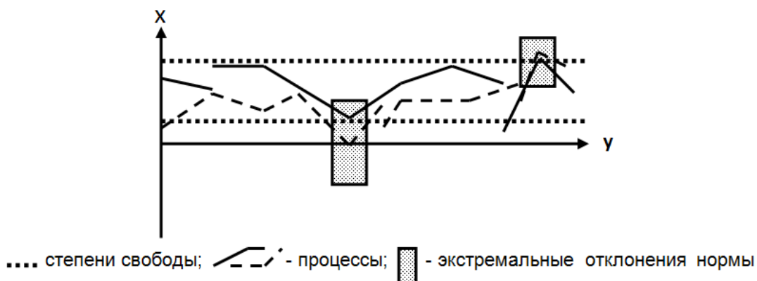
Рис. 2. Иллюстрация возможностей качественных изменений системы
