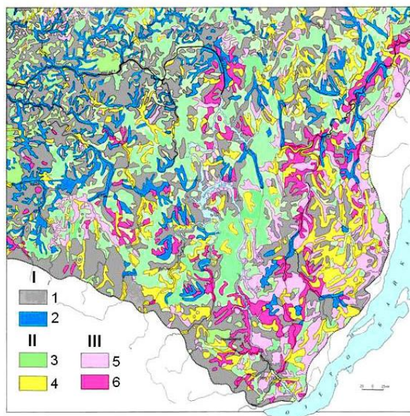
Рис. 3. Организация геосистем юга Средней Сибири. I-III – этапы процесса организации; 1-6 – подэтапы процесса организации. I –развитие: 1 – совершенствование взаимосвязей; 2 – сохранение и восстановление геосистемы без изменения ее свойств и цели; II – поддержание организации: 3 – замена старых подсистем на новые; 4 – изменение внутренних взаимосвязей; III –зарождение: 5 – генерация двух геосистем; 6 – разрушение и формирование новых взаимосвязей.
