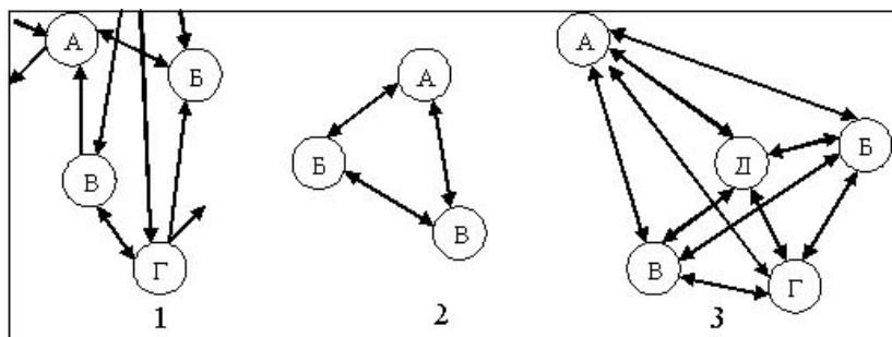
Рис. 1. Взаимосвязи частей геосистем. Типы взаимосвязей: 1 – дискретный, в котором элементы и подсистемы слабо взаимосвязаны между собой – экотоны и «молодые» системы; 2 – жесткие – серийные факторальные и реликтовые геосистемы; 3 – гармоничная согласованность разнообразных подсистем (коренные и многокоренные типы). А – Д – условные символы элементов системы. Стрелки - направления связей.
