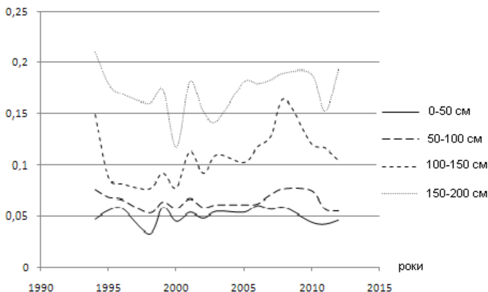
Рис.1. Динаміка засоленості ґрунтів Мічуринської рисової системи
